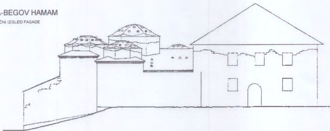
Crtež Isa-begovog hamama iz projekta zaštite i revitalizacije Stare čaršije u Novom Pazaru
