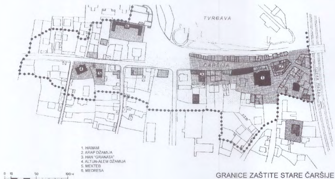
Crtež granica zaštite iz projekta zaštite i revitalizacije Stare čaršije u Novom Pazaru
