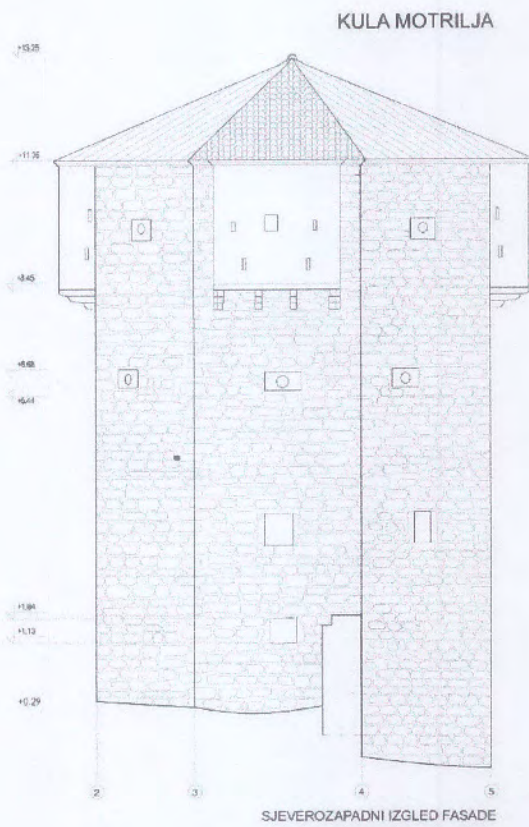
Crtež digitalizacije Kule Motrilje
